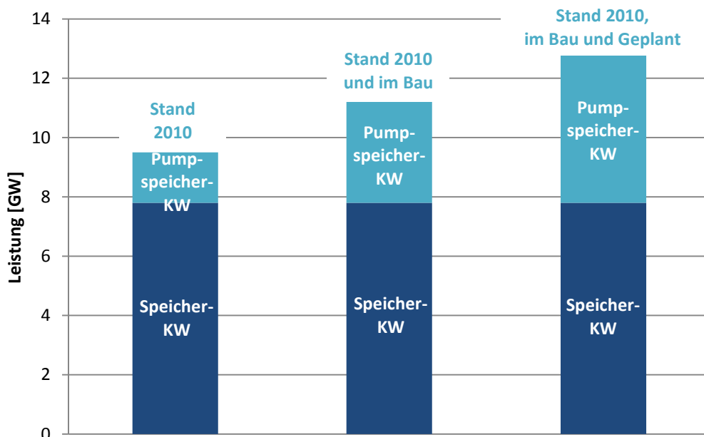
Abbildung 8: Schweizer Speicherkapazitäten & Ausbaupläne
