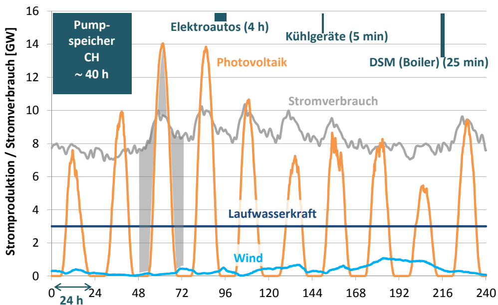
Abbildung 9: Möglichkeiten für aktives Lastmanagement in der Schweiz – PV und Windkraft aus Daten für Deutschland in der Periode 25.6.2011-3.7.2011, skaliert auf erwarteten Beiträge in der Schweiz im Jahr 2050 (Sommer, deswegen ohne Berücksichtigung von Wärmepumpen)
