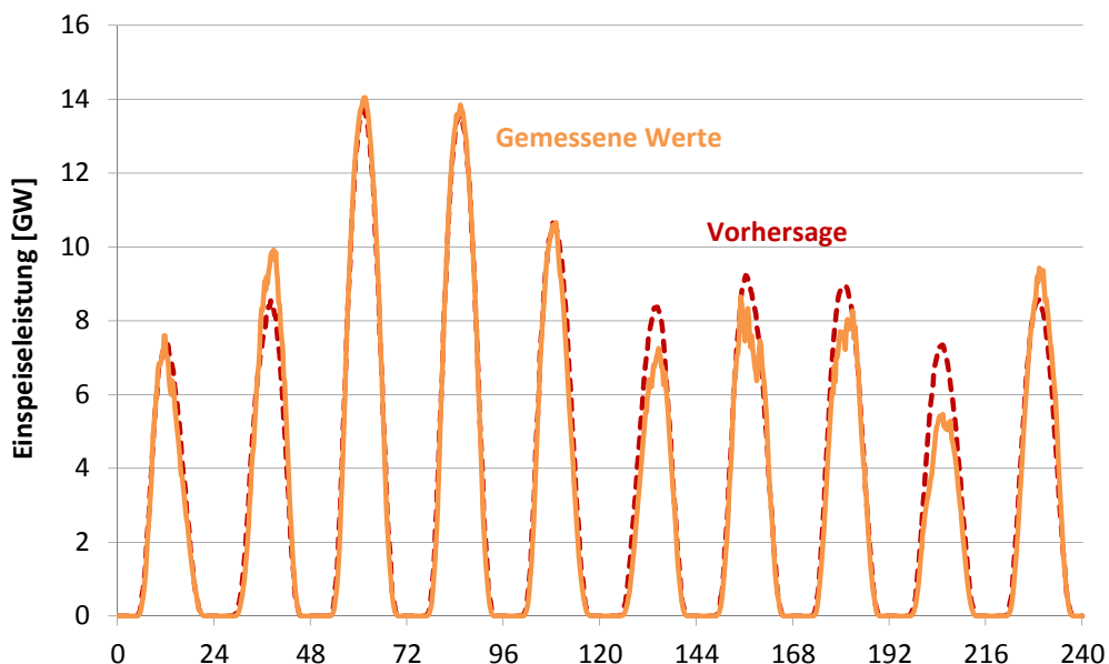
Abbildung 10: Energiemeteorologie für robuste Prognosen (PV-Erzeugung am Beispiel von Deutschland für die Periode 25.06.2011 bis 03.07.2011, skaliert auf erwarteten Beitrag im Jahr 2050)
