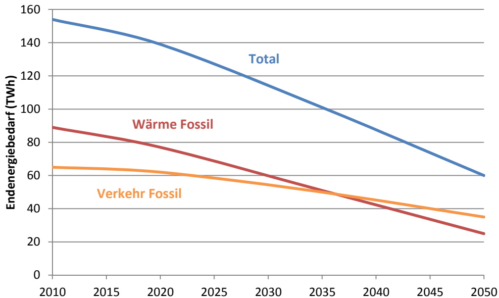
Abbildung 2: Absenkpfad der fossilen Energiemenge (Wärme, Mobilität und insgesamt, jedoch ohne fossile Stromproduktion) zur Erfüllung der Klimaziele.
