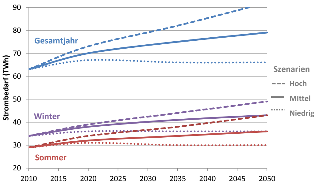
Abbildung 4: Strombedarf in der Schweiz – „Szenarien“ inkl. Netzübertragung, ohne Speicherpumpen, inkl. Zusatzstrom für Wärmepumpen und Mobilität
