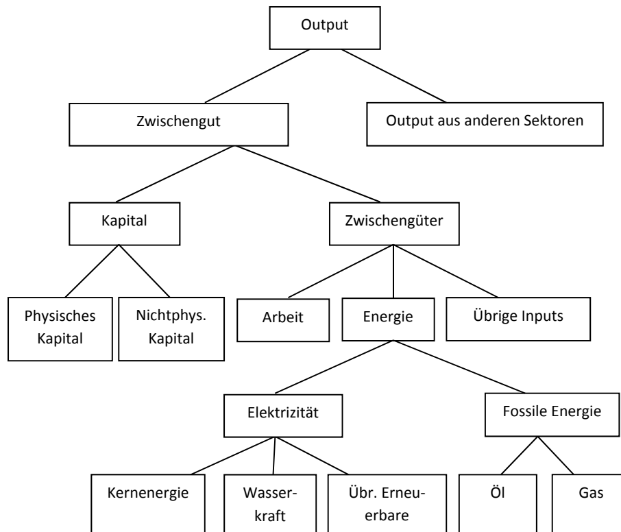
Abbildung 16: Schematische Darstellung der Produktion in einem Sektor (CITE-Modell), [68, 72]
