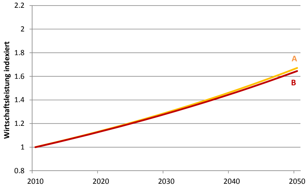
Abbildung 17: Vergleich von zwei Konsumpfaden 2010-2050; Pfad A mit Klimapolitik (obere Kurve in orange), Pfad B mit Klimapolitik und etappenweisem Ausstieg aus der Kernenergie (untere Kurve in rot)
