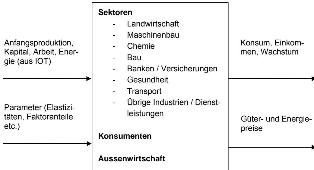
Abbildung 15: Input und Output im CITE-Modell [68, 69]
