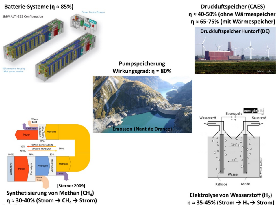
Abbildung 7: Optionen für die Stromspeicherung
