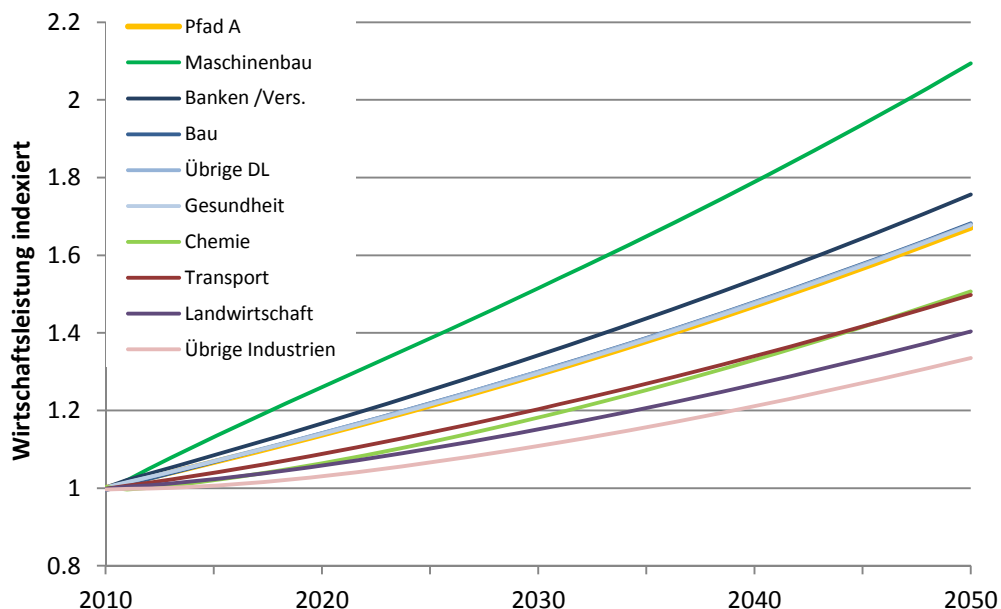
Abbildung 18: Branchenentwicklung mit Klimapolitik und etappenweisem Ausstieg aus der Kernenergie im Vergleich zu Pfad A aus Abb.17
